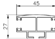
Standard-Doppelführungsschiene
