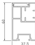
Distanz Führung ZS 60
