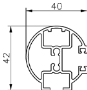
wie EF20 als runde Ausführung
