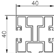
Verstärkte Führungsschiene für hohe Stabilität oder freitragende Ausführung
