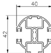
wie DF40 als runde Ausführung
